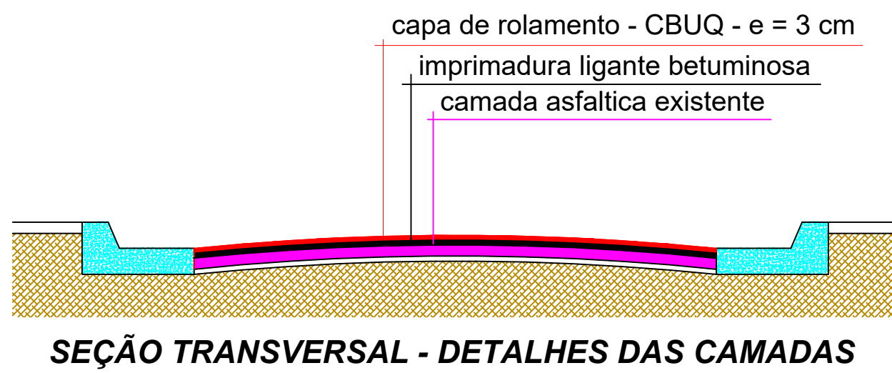
Detalhe 01 - Recapeamento Asfáltico (CBUQ)
