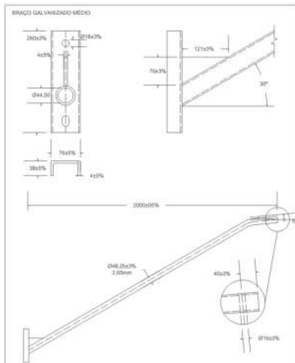
Figura 1 – Braço galvanizado de 2 metros.
